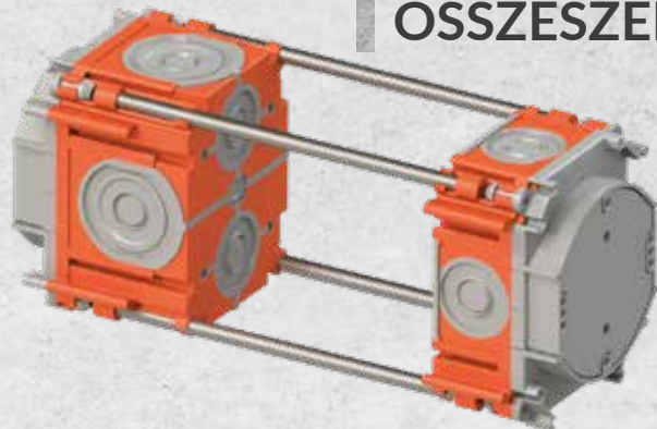
Példa a kétoldalú kötődobozok felszerelésére egy 6 mm átmérőjű acélrúd segítségével
