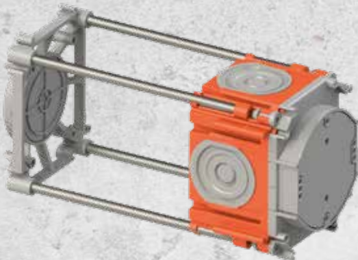
Példa a doboz rögzítésére a támaszték rendszer valamint 6 mm átmérőjű acélrudak segítségével
